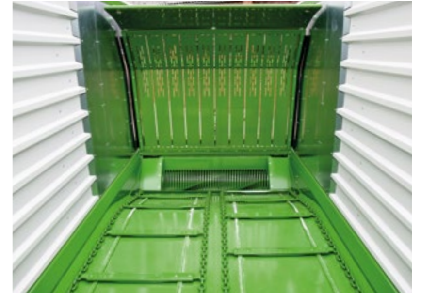
Abgesenkter Transportboden, 4 Ketten (je 14 x 50 mm, 25 t/Kette)
