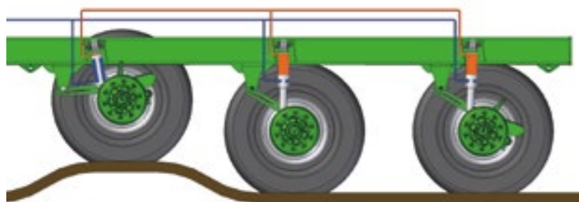
Tandem- und Tridem-Ausführung mit hydraulischem Fahrwerk
